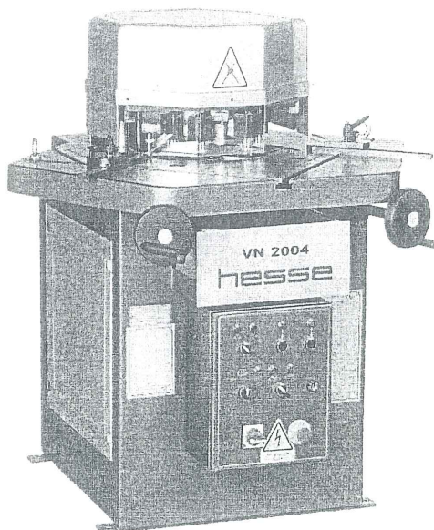
Slika 2. Stroj za isijecanje limova s podesivim kutom
