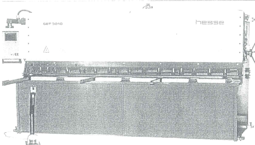
Slika 1. Hidraulički sjekač limova
