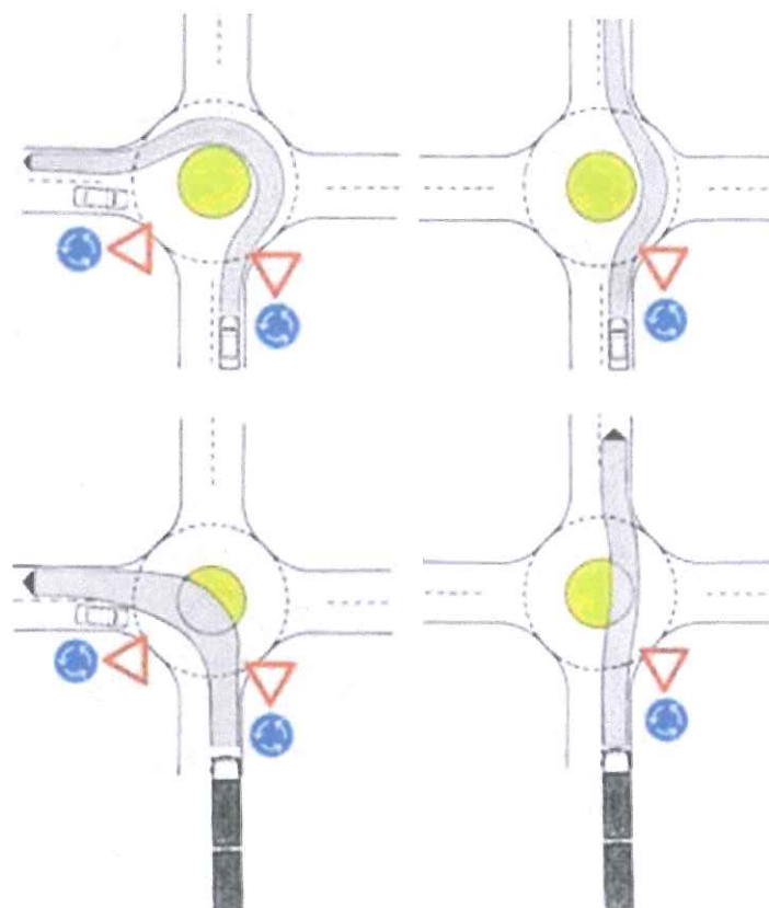
Skica prolaska osobnog i teretnog vozila kroz mini kružno raskrižje
