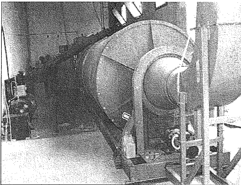
Rotacijska sušara za siječku
